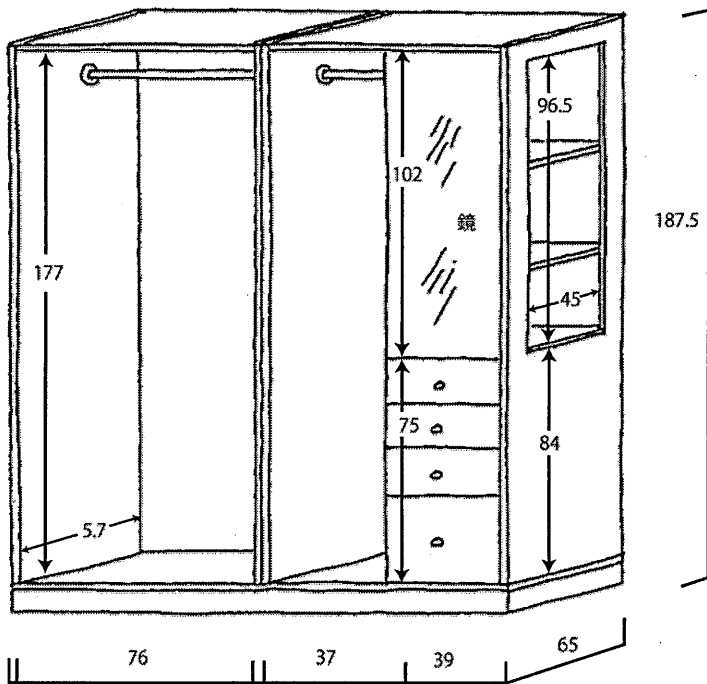
B館 クローゼット(扉 省略)
